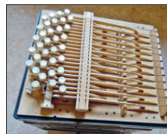
Mechanik der Tasten des Bandoneons
